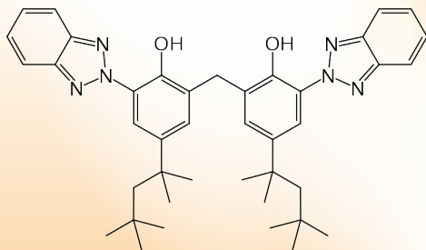
Tinosorb M的分子结构
